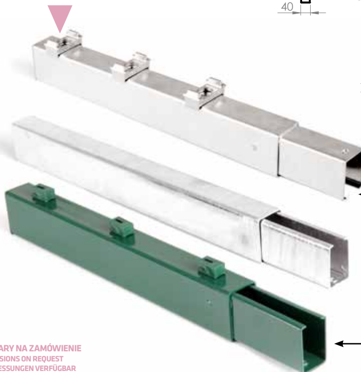
TYP A / TYPE A
