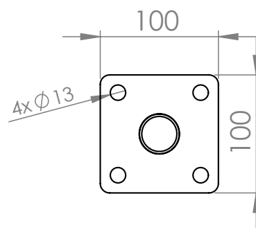
SŁUP Φ38 POST Φ38 >> PFOSTEN Φ38
