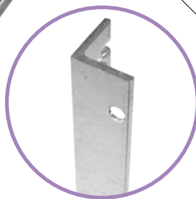
Kątownik 40x40x5 Kątownik 40x40x5 Winkelprofil 40x40x5 mm
