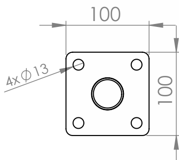
SŁUP Ø42 POST Ø42 >> PFOSTEN Ø42
