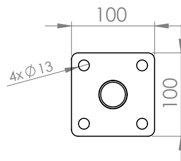
SŁUP Ø38 POST Ø38 >> PFOSTEN Ø38
